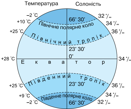
Мал. 5. Зональний розподіл солоності й температури вод Світового океану
