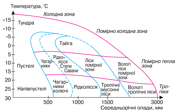
Мал. 2. Розподіл рослинно-тваринних угруповань залежно від кліматичних умов
