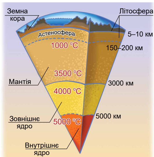
Мал. 1. Внутрішня будова Землі
