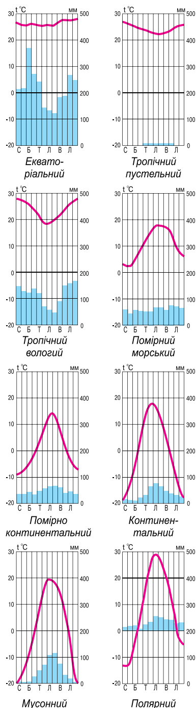
Малюнок. Кліматодіаграми річного ходу температур і опадів у різних кліматичних поясах Землі
