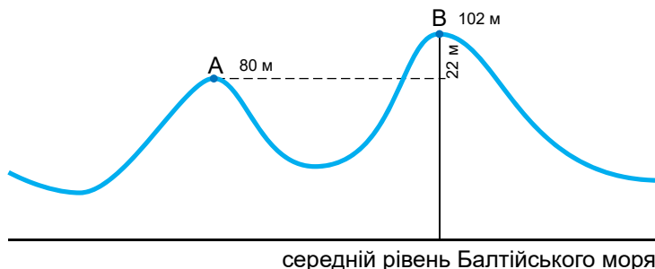
Мал. 9. Абсолютна та відносна висота місцевості
