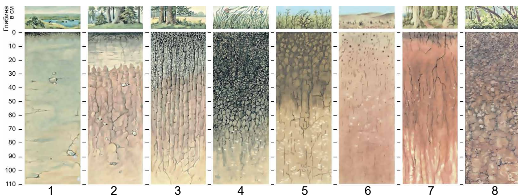
Малюнок. Профілі різних ґрунтів Землі:
