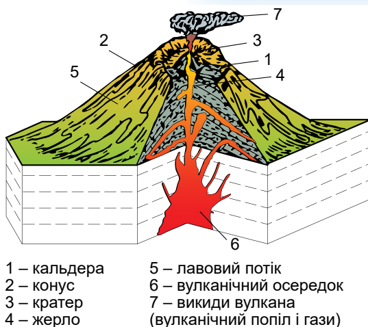
Мал. 1. Схема будови вулкана
