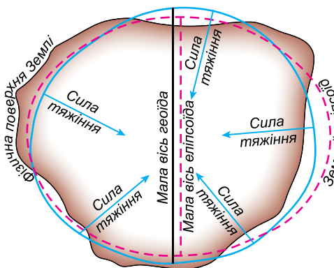
Мал. 1. Геоїд та земний еліпсоїд
