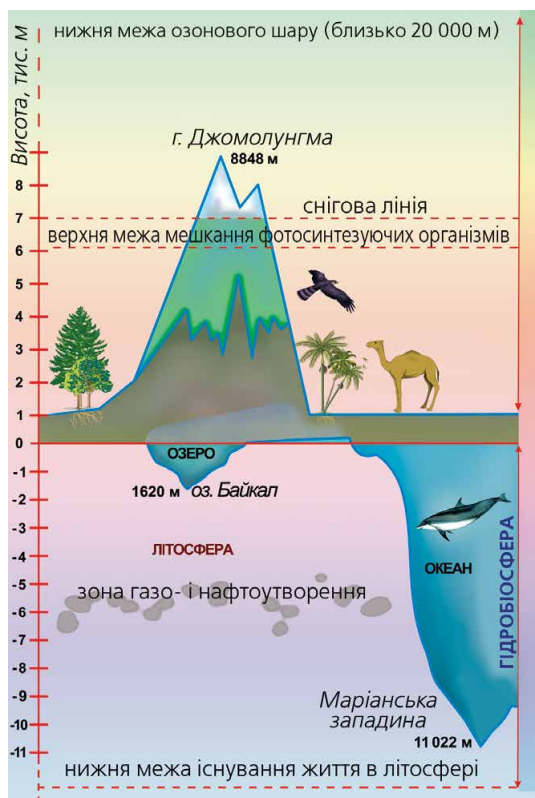
Мал. 1. Межі біосфери
