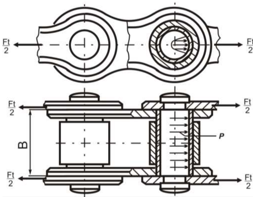
Рисунок 9.5 – Розрахункова схема
