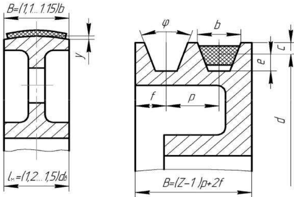
Рисунок 10.8 – Конструкції шківів
