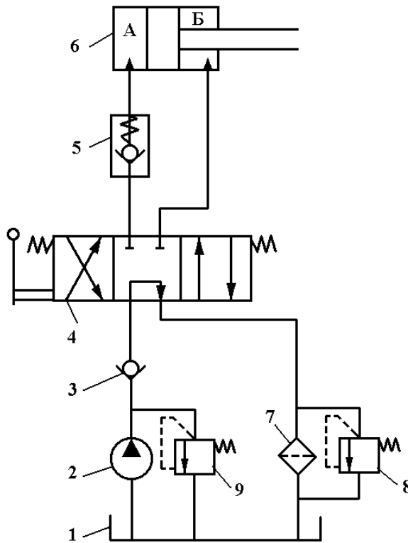
Рисунок 32.10 – Схема гідравлічна одноплунжерного підіймача
