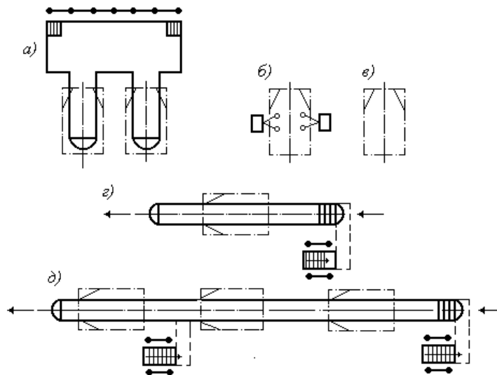
а), б), в) – тупикові: з канавою, з підйомачем, підлоговий; г) – проїзний з канавою; д) – спеціалізовані на лінії з канавою
