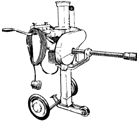
Рисунок 34.2 – Загальний вигляд електромеханічного інерційно-ударного гайковерта для гайок коліс автомобіля
