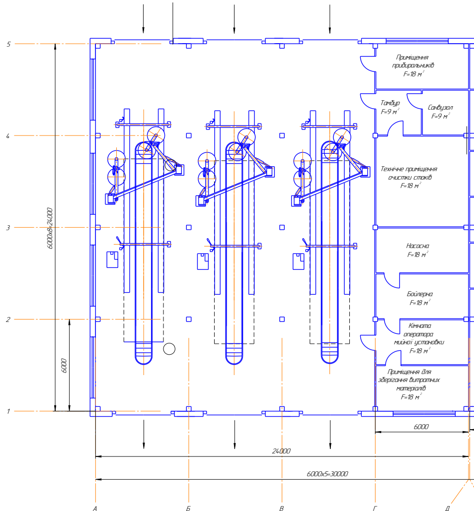
Рисунок 10.5 – Зона ЩО для обслуговування автобусів
