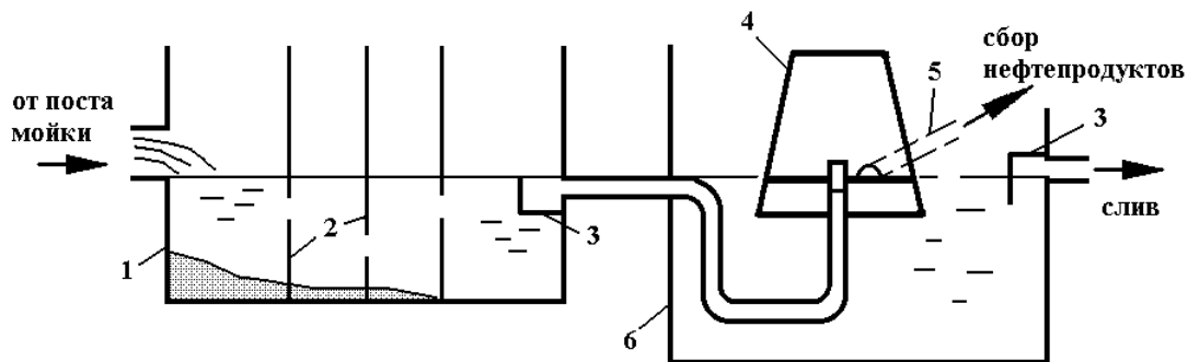
1 – корпус відстійника; 2 – заспокоювачі води; 3 – відбійник; 4 – ковпак; 5 – трубопровід; 6 – корпус маслобензовловлювача.
