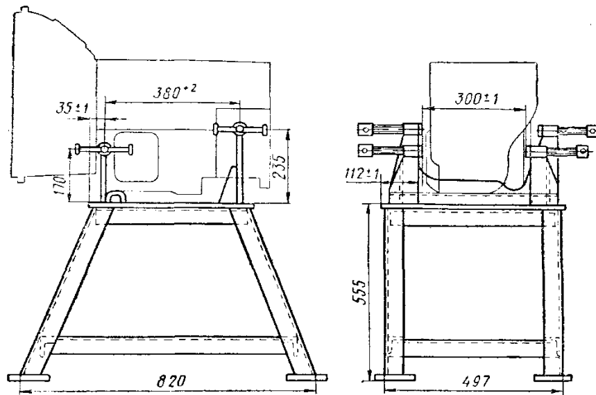
Рисунок 34.5 – Стенд для розбирання та збирання коробок передач
