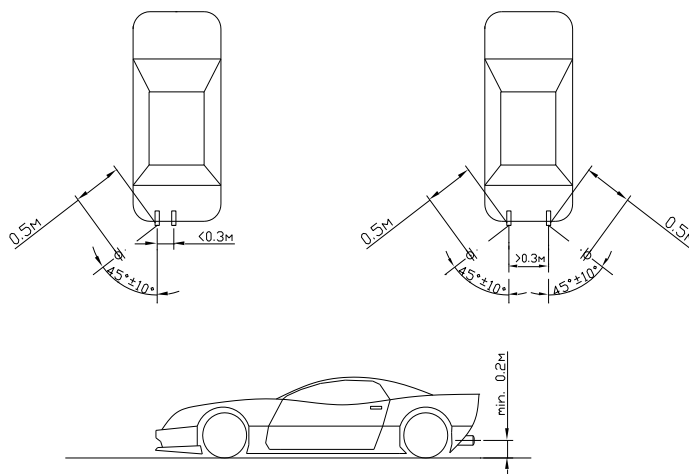
Рисунок 11.4 – Проведення випробувань нерухомого КТЗ, розташування мікрофона шумоміра за наявності декількох вихлопних труб.
