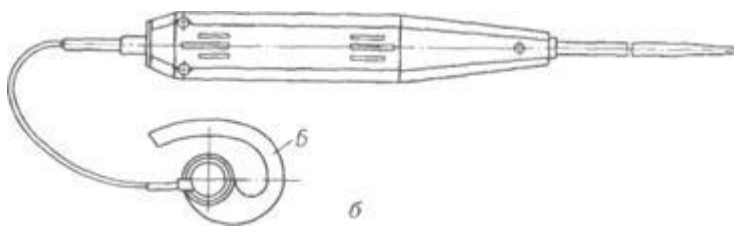
Рисунок 11.1 – Стетоскопи: а) найпростіший КИ-1154; б) електронний: 1 – привід; 2 – елементи живлення; 3 – корпус-ручка; 4 – перетворювач; 5 – стержень; 6 – телефон-навушник
