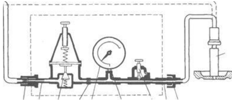
Рисунок 11.8 – Прилад К-69М: 1 – муфта швидкознімна; 2 – штуцер вхідний; 3 – редуктор; 4 – сопло вхідне; 5 – манометр вимірювальний; 6 – демпфер; 7 – гвинт регульовальний; 8 – штуцер вихідний; 9 – сполучна муфта; 10 – штуцер
