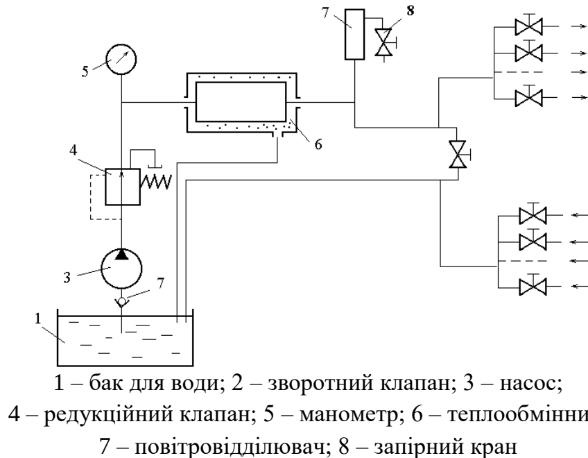
Рисунок 36.2 – Схема підігріву гарячою водою
