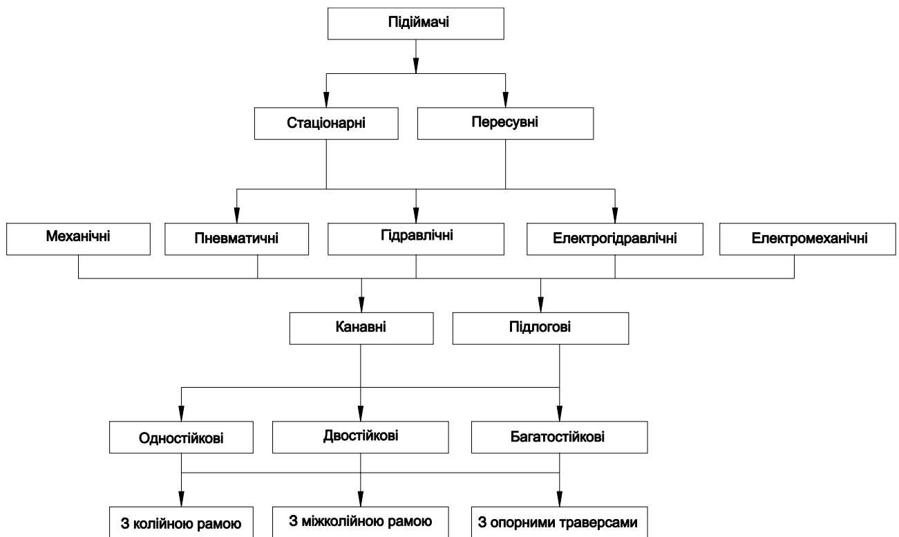
Рисунок 32.4 – Класифікація підйомних пристроїв, застосовуваних при ТО і ремонті автомобілів
