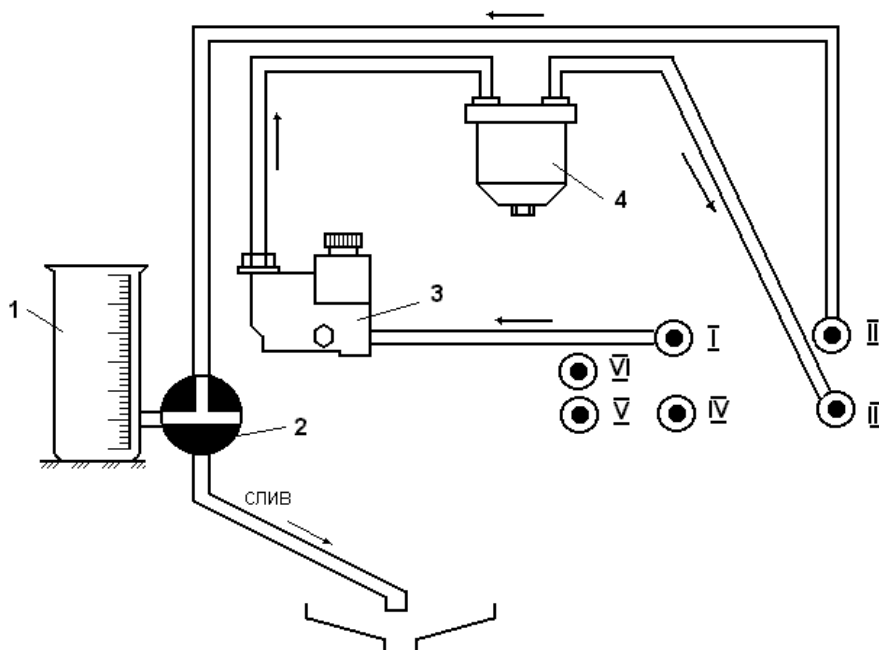
1 – мірний циліндр; 2 – триходовий кран; 3 – насос; 4 – випробуваний фільтр Рисунок 18.4 – Схема з'єднань паливопроводів при діагностуванні фільтрів
