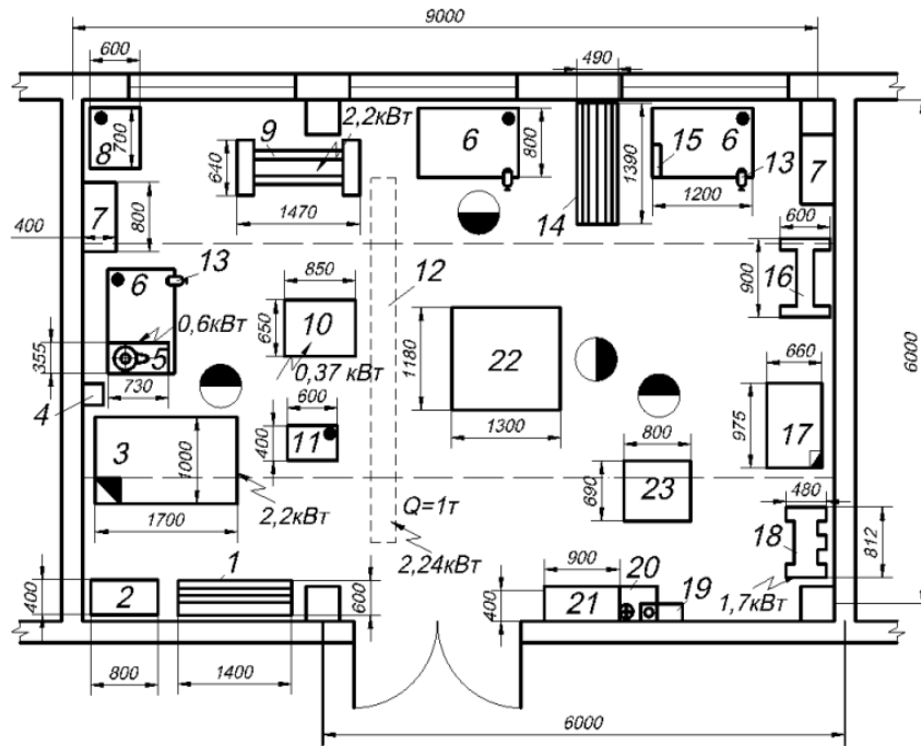
1 – стелаж для деталей; 2 – скриня для ганчір'я; 3 – верстат для розточування гальмових барабанів; 4 – телефон і радіо; 5 – настільний свердлильний верстат; 6 – слюсарний верстак; 7 – настінна шафа для приладів і інструментів; 8 – стенд для розбирання і регулювання зчеплень; 9 – гідравлічний прес 40 т; 10 – стенд для ремонту редукторів задніх мостів; 11 – стенд для клепання гальмівних накладок; 12 – підвісна кран-балка; 13 – лещата; 14 – стелаж для інструментів; 15 – настільний прес на підставці; 16 – стенд для ремонту карданних валів і рульових механізмів; 17 – миюча ванна для деталей; 18 – заточувальний верстат; 19 – електричний рукосушитель; 20 – умивальник; 21 – скриня для відходів; 22 – стенд для ремонту передніх і задніх мостів; 23 – стенд для ремонту коробок передач. Рисунок 41.2 – Агрегатне відділення АТП вантажних автомобілів
