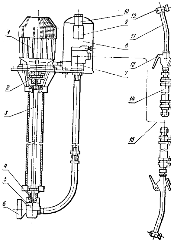
1 – електродвигун; 2 і 4 – муфти; 3 – приводний вал; 5 – насос; 6 – фільтр; 7 – блок клапанів; 8 – повітряно-гідравлічний акумулятор; 9 – реле тиску; 10 – манометр; 11 – роздатковий стовбур; 12 - відсічний клапан; 13 – запірний клапан; 14 – роздатковий рукав; 15 – маслопровід
