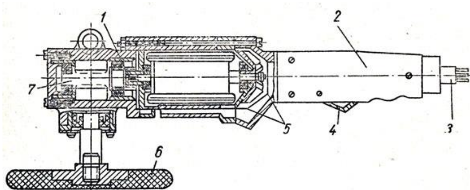
Рисунок 21.5 – Прилад для полірування кузовів автомобілів (модель 2408): 1 - муфта; 2 - рукоятка; 3 - кабель; 4 - пусковий курок; 5 - електродвигун; 6 - диск; 7 - черв'як редуктора
