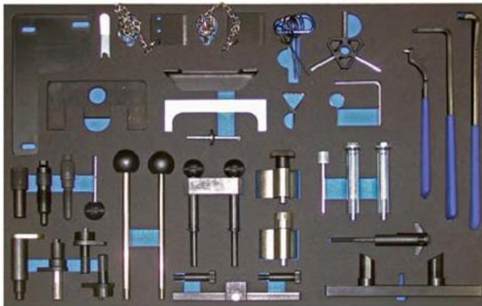
Рисунок 34.12 – Набір для обслуговування двигунів VW-Audi
