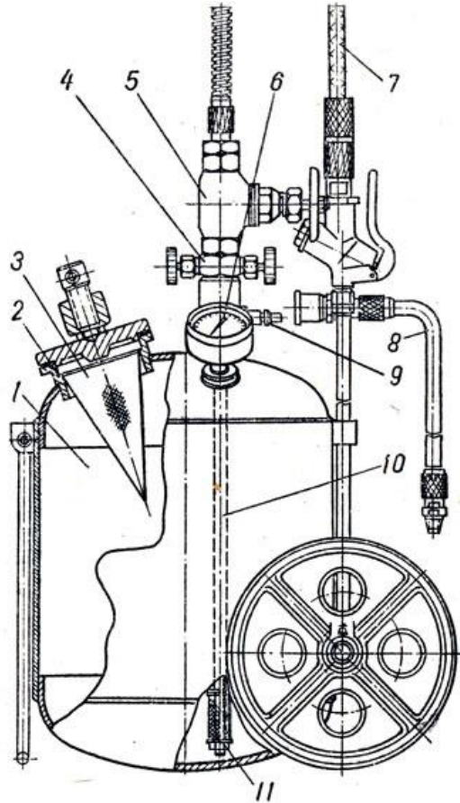
Рисунок 21.4 – Установка для нанесення антикорозійного покриття (модель 183 - 1)
