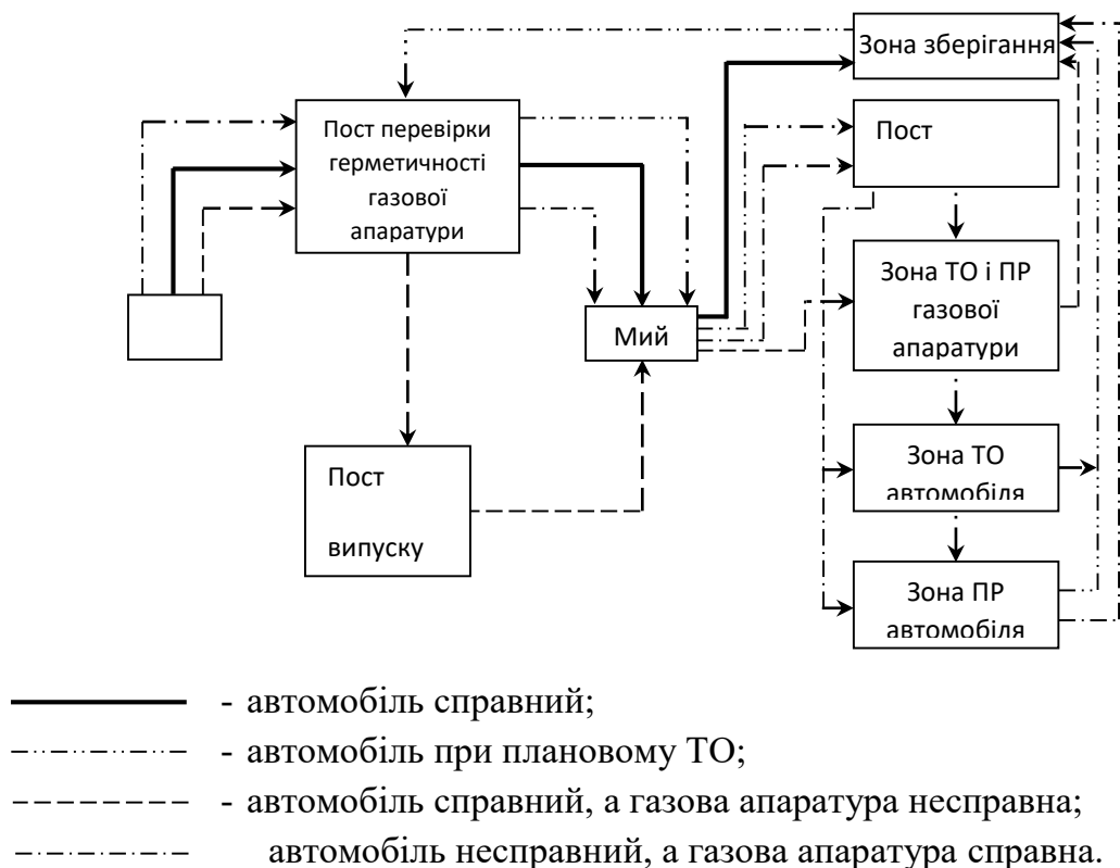
Рисунок 19.1 Схема технологічних процесів ТО і ПР газобалонних автомобілів, які працюють на СПГ
