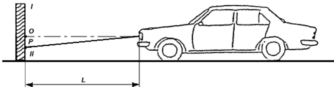
Рисунок 20.3 – Першочерговий кут нахилу фар.
