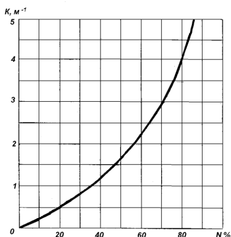
Рисунок 12.5 – Графік переведення коефіцієнта ослаблення світлового потоку N , % у натуральний показник ослаблення світлового потоку K , \text{м}^{-1}
