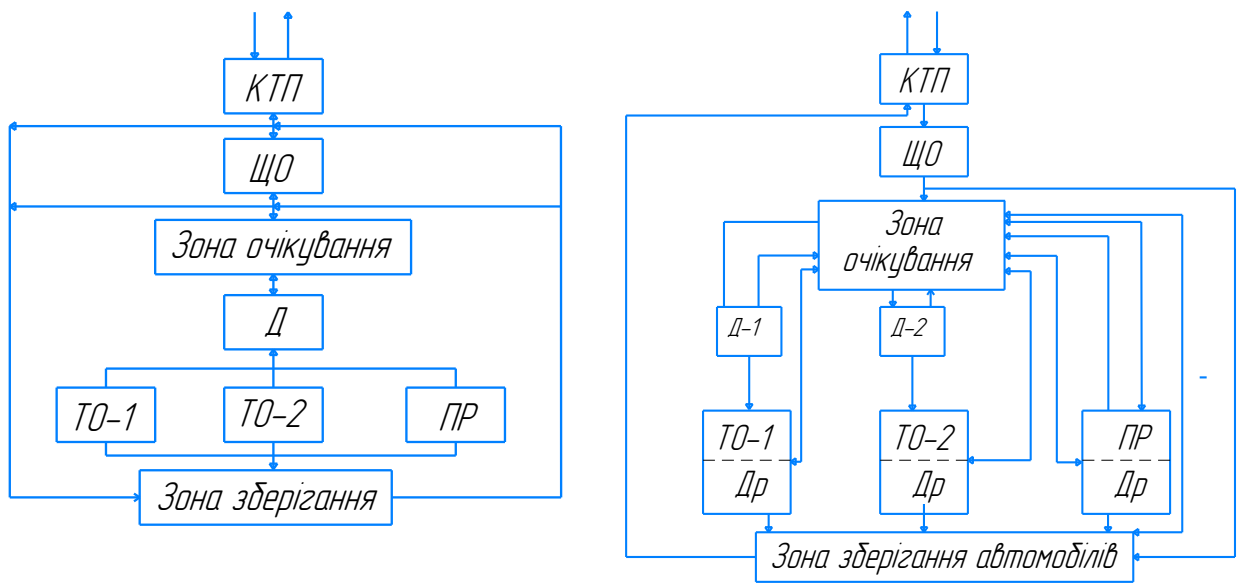
Рисунок 25.1 – Можливі схеми організації процесів ТО і ремонту з діагностуванням
