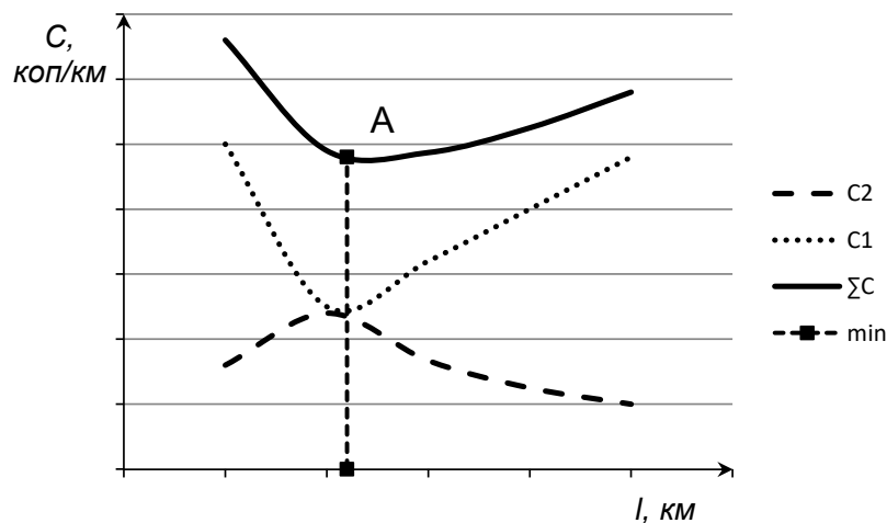
Рисинок 5.1 – Зміна витрат на технічне обслуговування і поточний ремонт у залежності від періодичності їх проведення
