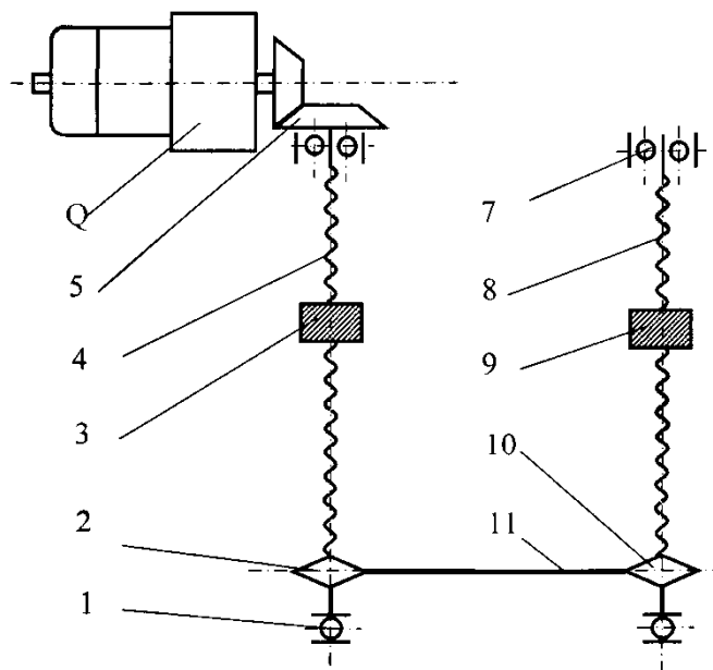
Рисунок 32.14 – Схема електромеханічного підіймача
