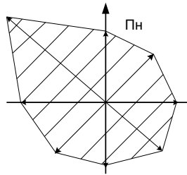
Рисунок 39.2 – Троянда вітрів
