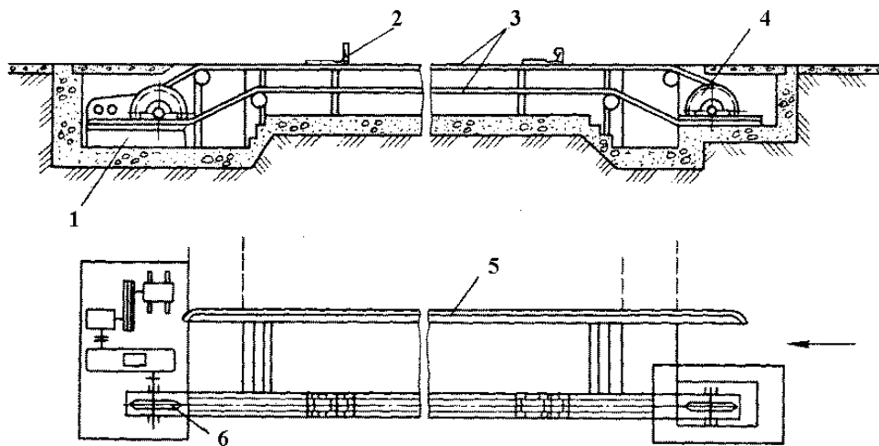
Рисунок 3.20 – Схема штовхаючого конвеєра
