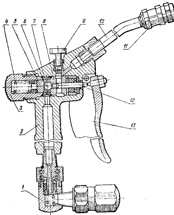
1- шарнір; 2 – корпус; 3 – заглушка; 4 – пружина; 5 – гніздо клапана; 6 – клапан; 7 – розподільне кільце; 8 – гільза; 9 – гвинт скидання тиску; 10 – стовбур; 11 – мастильна головка; 12 – плунжер; 13 – важіль
