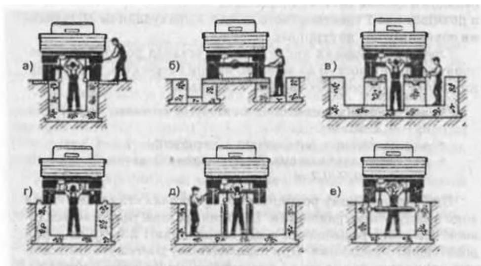
Рисунок 32.1 – Оглядові канали: а) міжколійна; б) бічна; в) комбінована; г) міжколійна із зовнішніми ребордами; д) комбінована механізована; е) міжколійна механізована
