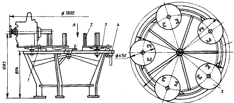
1 – поворотний стіл; 2 – кронштейн для установки коробок передач; 3 – поворотні диски; 4 – стопорний пристрій
