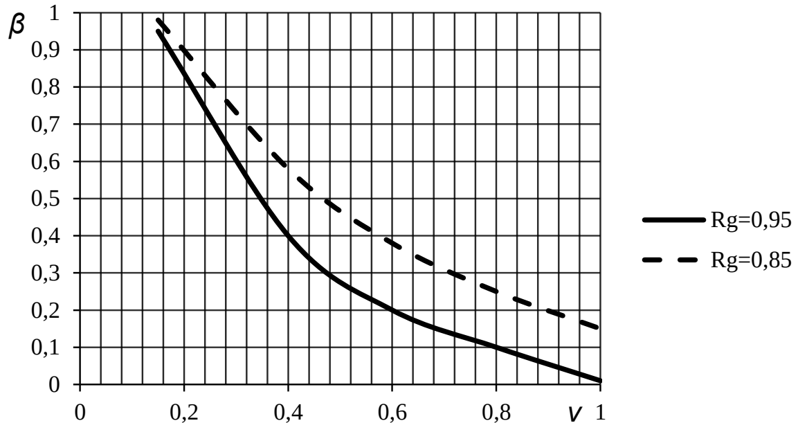
Рисунок 5.2 – Графіки для визначення \beta залежно від рівня безвідмовності та коефіцієнта варіації v .
