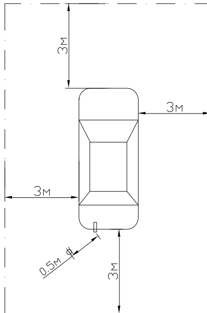
Рисунок 11.3 – Проведення випробувань нерухомого КТЗ, розташування мікрофона шумоміра.
