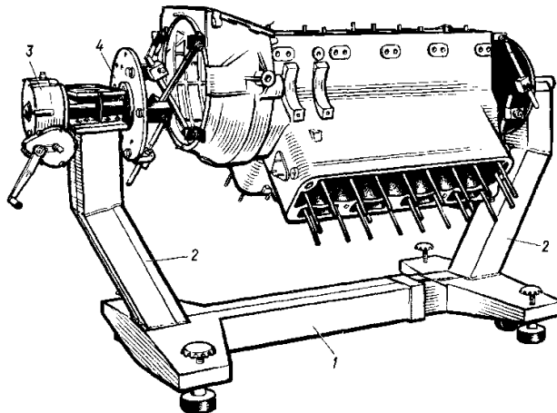
Рисунок 34.4 – Загальний вигляд стенду-кантувача для розбирання та збирання двигуна
