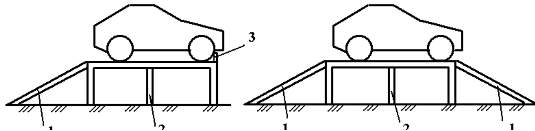
Рисунок 32.3 – Схеми естакад
