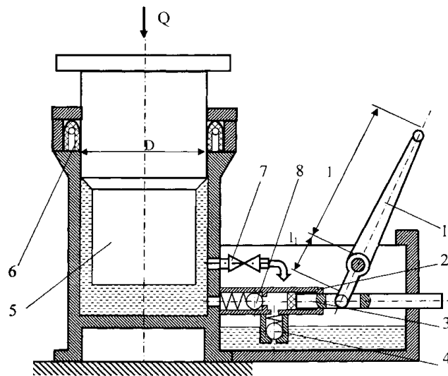
Рисунок 32.7 – Схема гідравлічного домкрата
