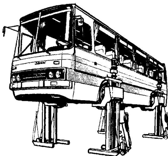
Рисунок 32.15 – Підіймач – комплект пересувних стійок для вантажних автомобілів і автобусів
