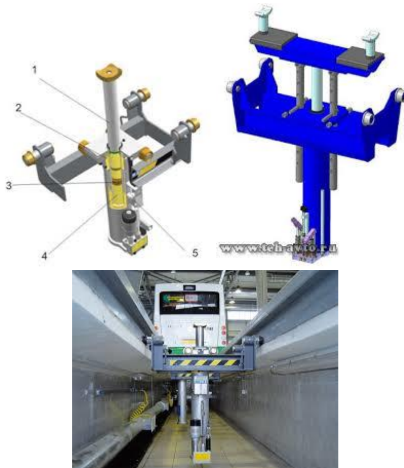
Рисунок 32.17 – Канавні підіймачі
