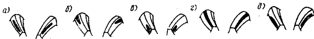
Рисунок 22.2 – Зсув плями контакту на зубах веденої шестерні головної передачі
