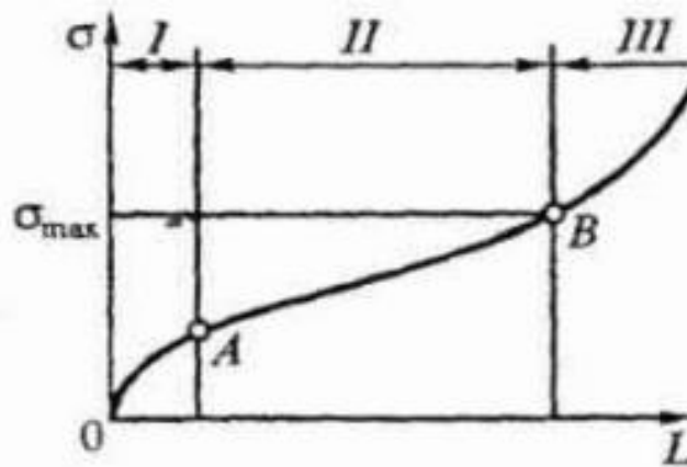
Рисунок 2.1 – Залежність спрацювання та інтенсивності спрацювання деталей автомобіля від його пробігу (для сталих умов експлуатації)
