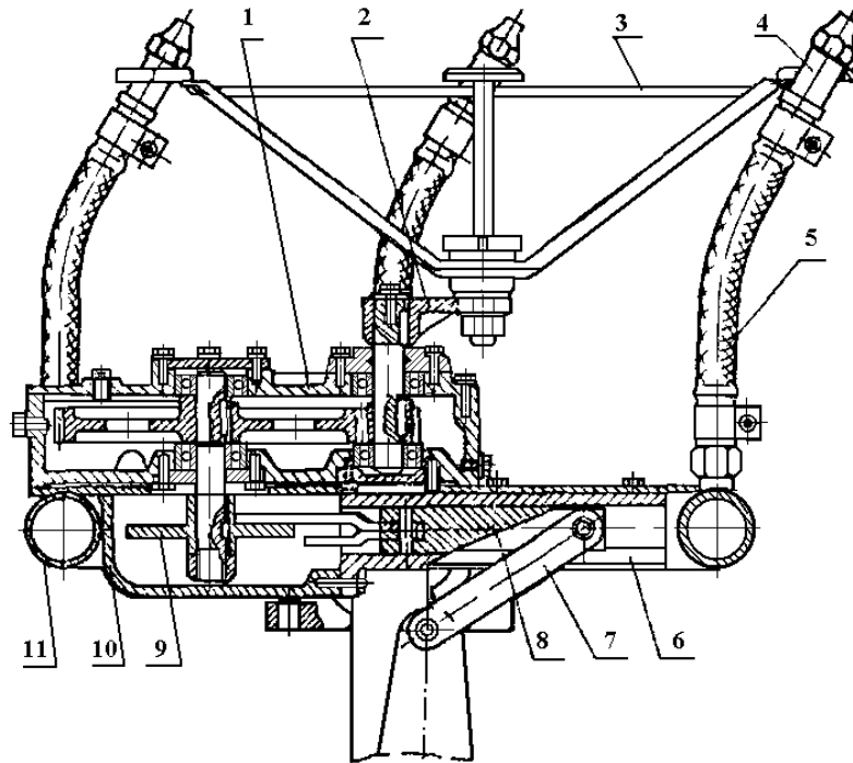
1 - редуктор; 2 і 7 - важелі; 3 - повідкове кільце; 4 - соплова насадка; 5 - шланг; 6 - напрямна повзуна; 8 - повзун; 9 - храпове колесо; 10 - кришка; 11 - колектор
