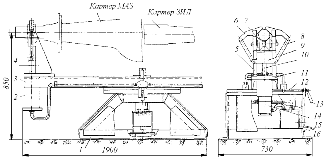
Рисунок 34.7 – Стенд для кріплення картера ведучого моста
