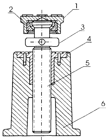
Рисунок 32.5 – Схема гвинтового домкрата
