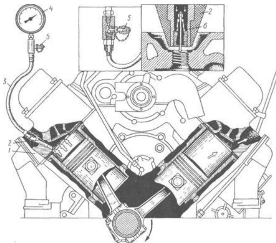
Рисунок 11.7 – Схема перевірки компресії: 1 – головка циліндрів; 2 – гумовий наконечник; 3 – шланг; 4 – манометр; 5 – клапан випуску повітря; 6 – золотник
