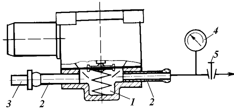
1 – вакуумна порожнину; 2 – патрубки; 3 – заглушка; 4 – вакууметр; 5 – кран Рисункок 19.4 – Схема перевірки герметичності вакуумної порожнини дозуючого-економізаторного пристрою
