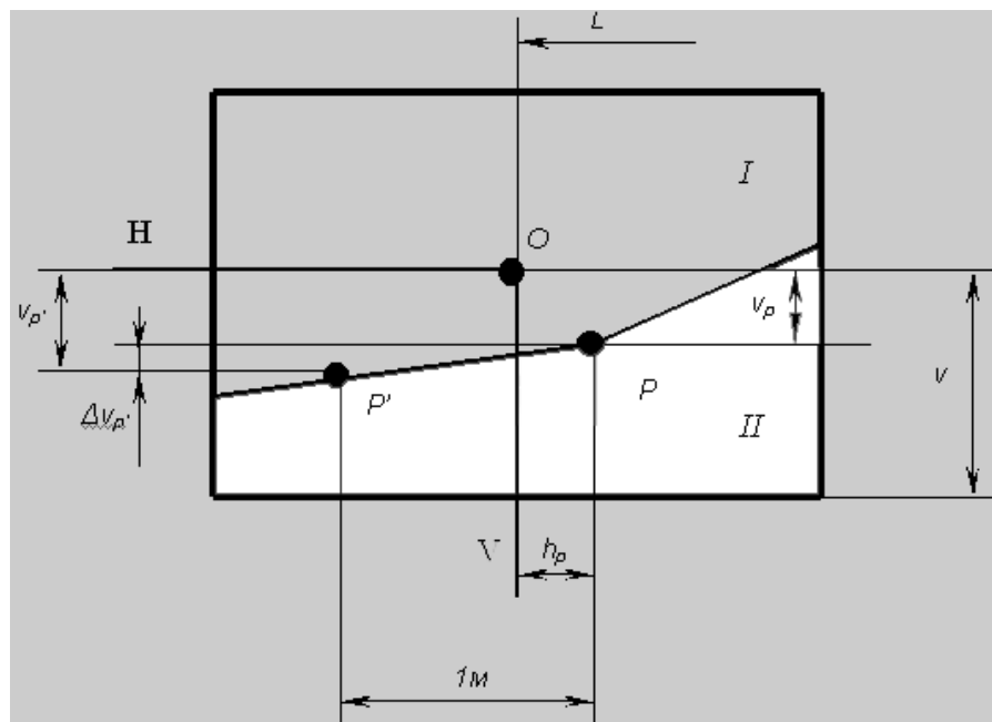
Рисунок 20.3 – Першочерговий кут нахилу фар.
