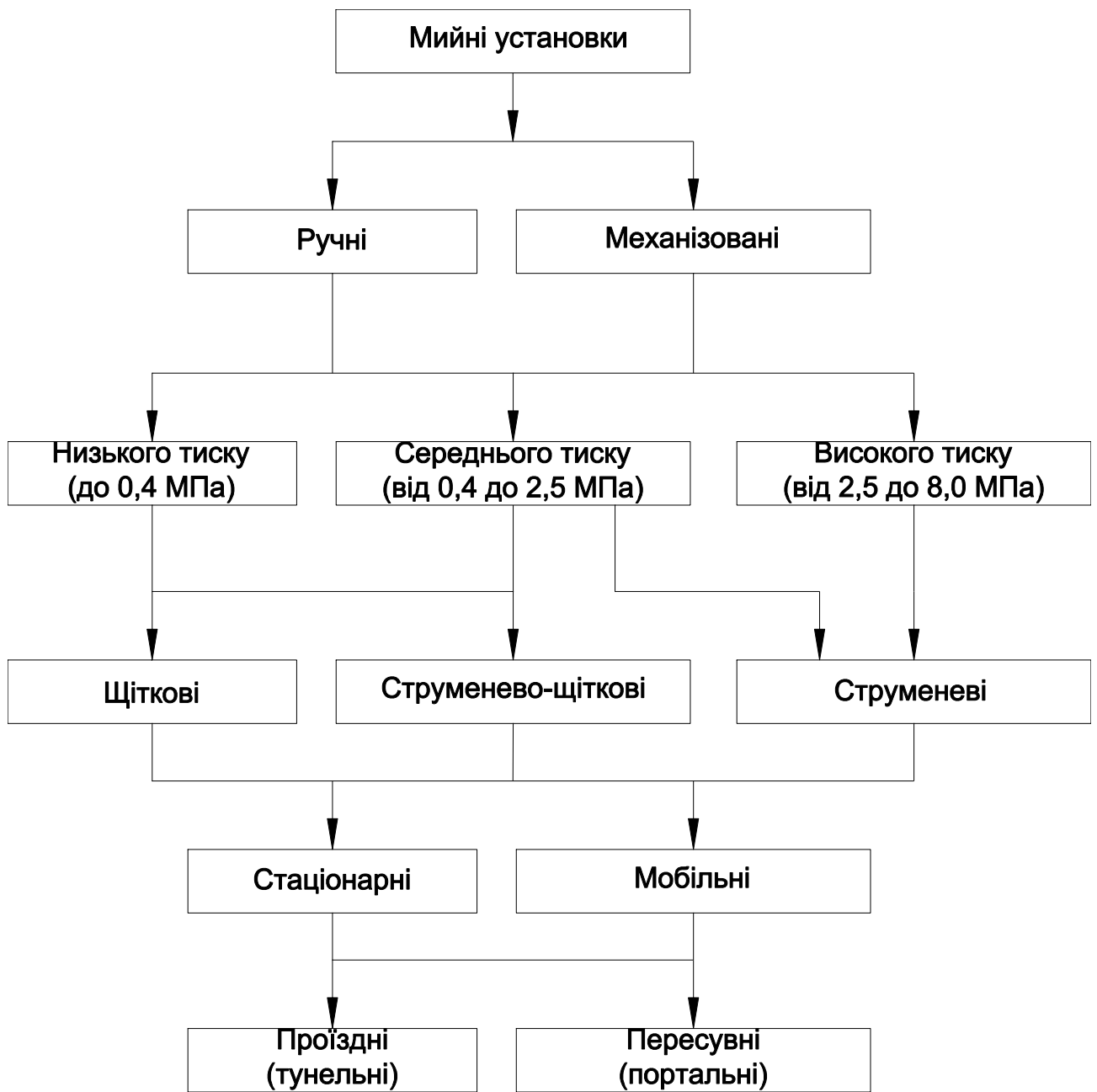
Рисунок 31.1 – Схема класифікації установок для зовнішнього миття автомобілів
